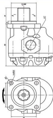
XPL外形及安装尺寸—XPL DIMENSIONS
