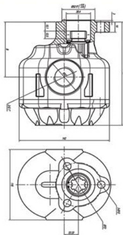
XP外形及安装尺寸—XP DIMENSIONS
