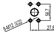
A, B 油口法兰
